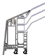
3-schalig U_g -Wert 1,8 U_r -Wert 1,6
