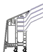
4-schalig U_g -Wert 1,5 U_r -Wert 1,3
