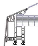
thermoplan U_g -Wert 0,83 U_r -Wert 0,83
