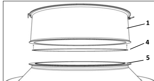
Bild 1: Montage Sanierungsaufsetzkranz
