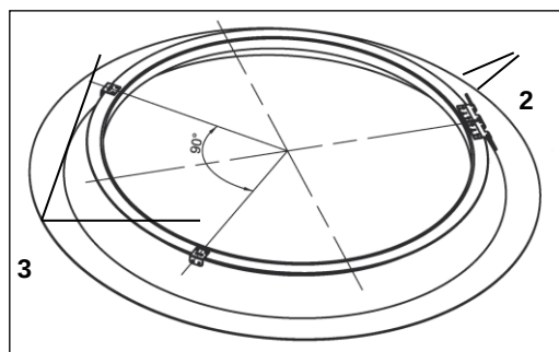
Bild 4: montierter esserfix® - tandem Aufsetzkranz
