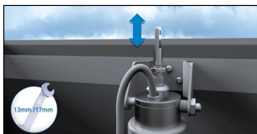
4 Augenschraube einstellen Adjust eyebolt
