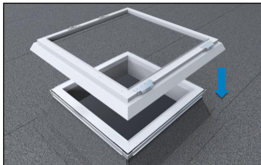
9 Sanierungsrahmen aufsetzen Put on renovation frame
