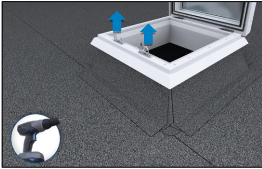
7 Schließbleche demontieren Demount striking plates
