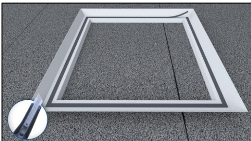
8 Dichtband einkleben Apply sealing tape
