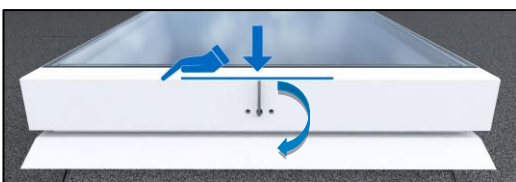
17 FDF herunterdrücken und durch 90°- Drehung des Vierkants verriegeln Gently press down the skylight and lock the flat glass skylight by turning the square shaft 90° clockwise
