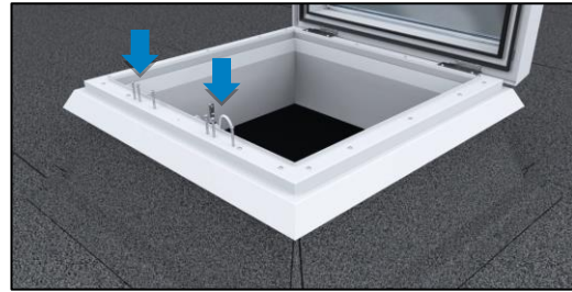
8 Löcher mit Schrauben verschließen Close holes with screws
