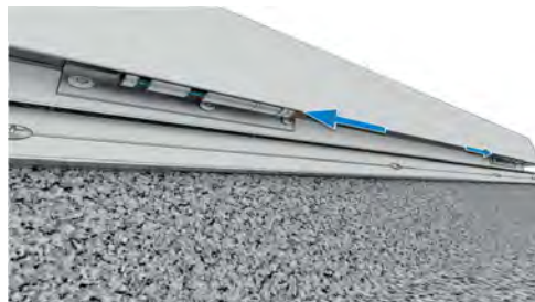
6.2 Scharnierbolzen einschlagen Drive in hinge bolts
