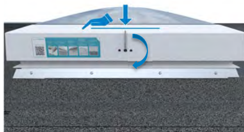
8 Lichtkuppel / FDF durch 90° Drehung des Vierkants verriegeln Lock the skylight by turning the square shaft 90° clockwise
