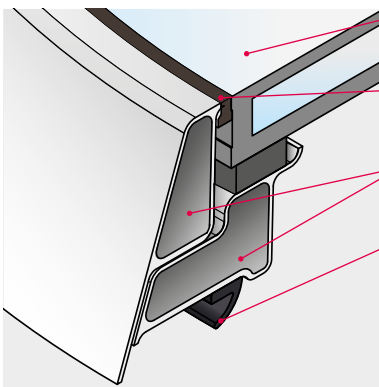
Wärmedämmverglasung ESG außen 2- oder 3-fach
