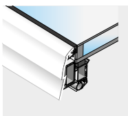
Wärmedämmverglasung 2-fach U-Wert 1,1 W/m 2 K
